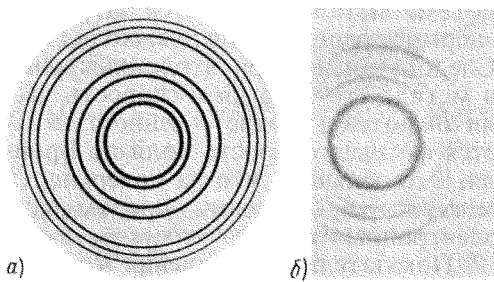
Электронogramмы листов серебра (а) и золота (б) в опытах Томсона и Тартаковского
