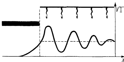
Интенсивность волны при дифракции на прямолинейном крае полубесконечной плоскости
