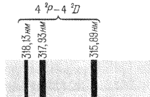
Спектр энергетических уровней калия с учетом мультиплетности
