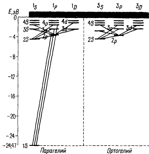
Энергетические уровни парагелия и ортогелия
