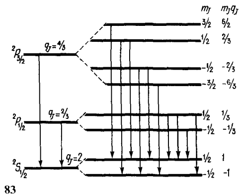
83 Расщепление энергетических уровней атома натрия, переходы между которыми обуславливают излучение главной серии
