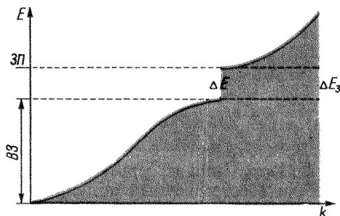
Энергетический спектр полупроводника
