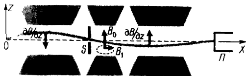
Схема опыта по наблюдению магнитного резонанса для измерения магнитного момента атома
