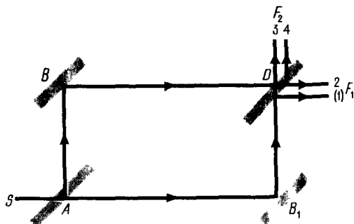
Схема интерферометра Маха-Зендера
