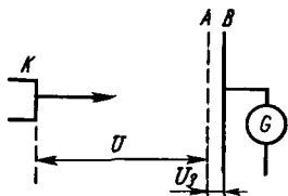
Схема опытов Франка – Герца
